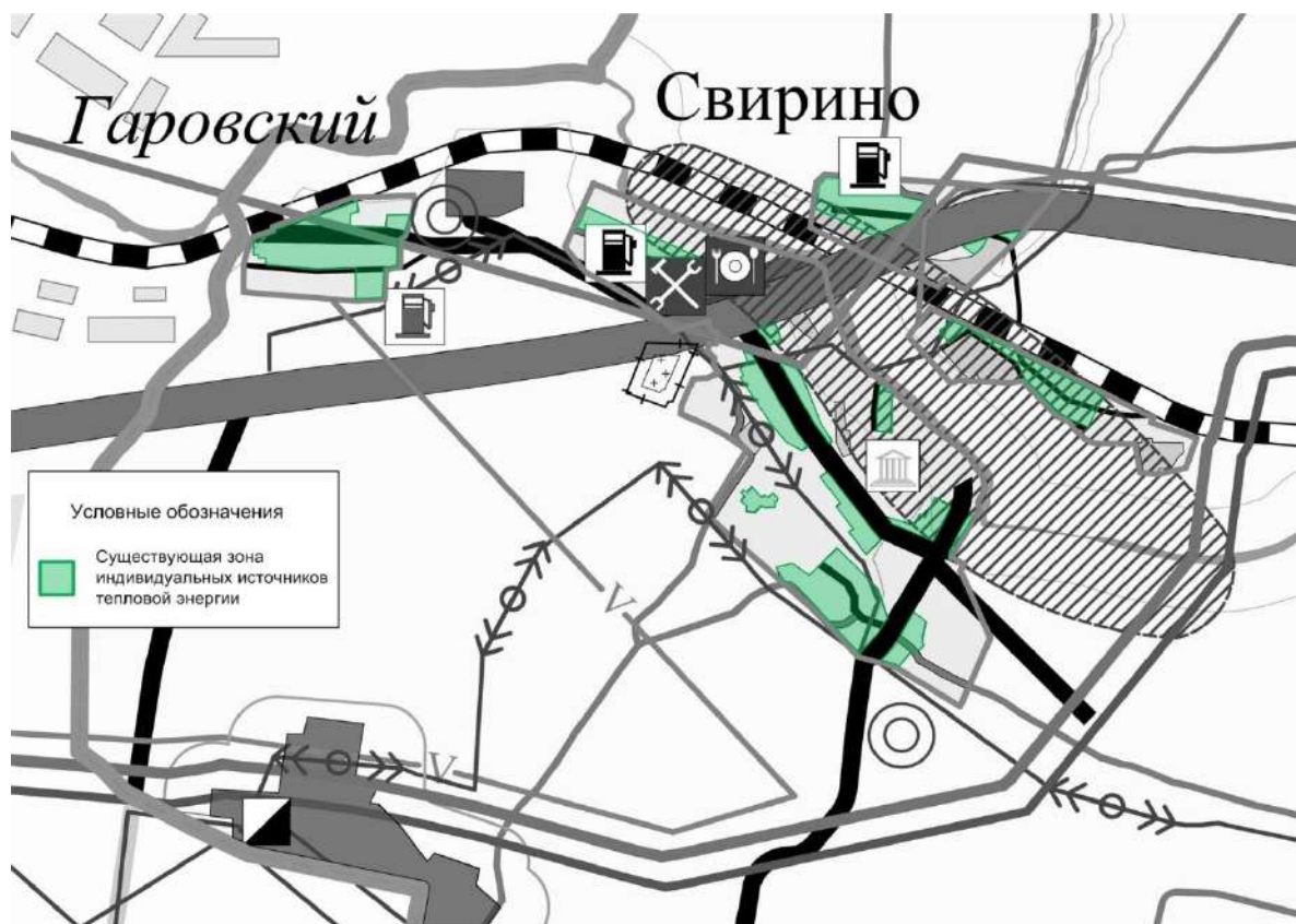
Рисунок 2.2.3 – Существующие зоны действия индивидуальных источников тепловой энергии с. Свирино и п. Гаровский
